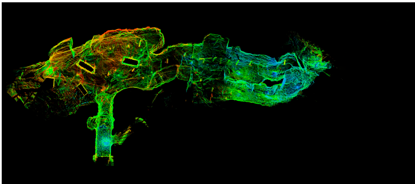
Planimetria della galleria aperta al pubblico della Pesciara, realizzata con il Laser-scanner (rilievo F. Dalle Pezze, 2015)
