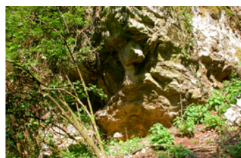
C. Ciupio. La parete rocciosa alla cui base si trovano gli strati fossiliferi, attualmente coperti da detrito.
