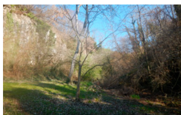
A. Panoramica della valletta con il corso d'acqua che ha inciso il giacimento
