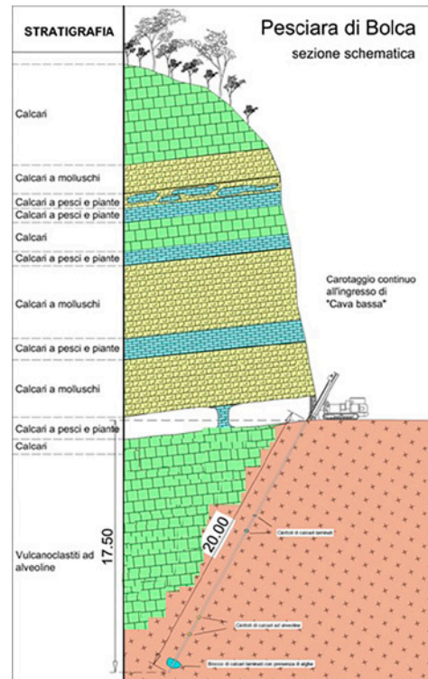
Pesciara: carotaggio continuo inclinato eseguito nel 2011 in prossimità dell'ingresso di una galleria scavata nell'800 e, a destra, sezione stratigrafica schematica.
