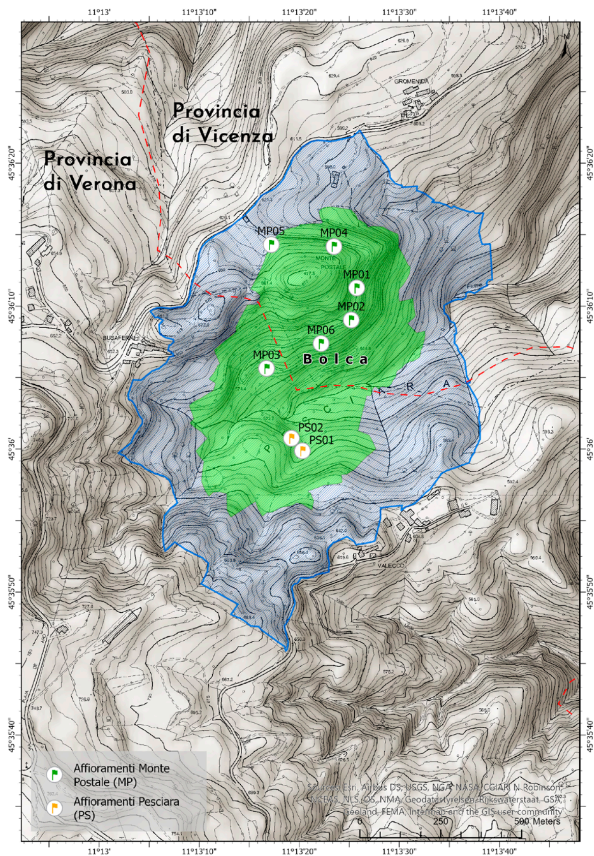
6.1.a Carta topografica della core zone e buffer zone della componente Bolca con gli affioramenti fossiliferi (Allegato 6 Cartografia, carta 6.1.a)
