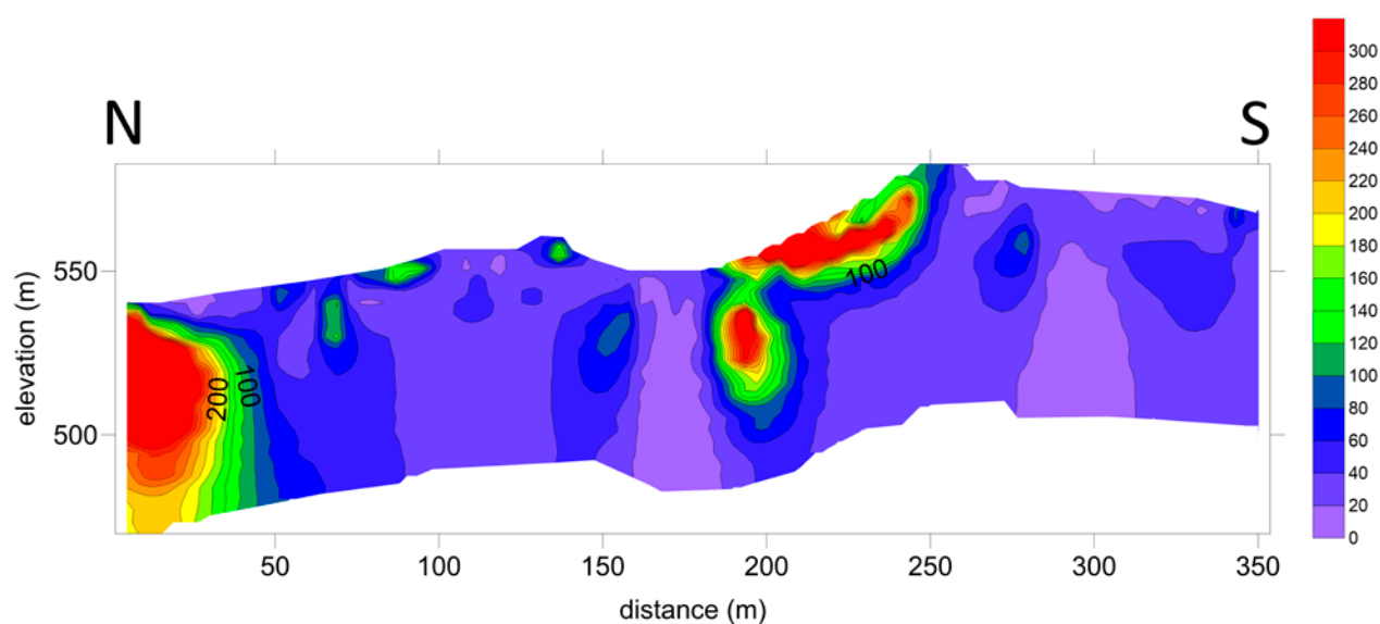
Profilo geoelettrico nell'area della Pesciara
