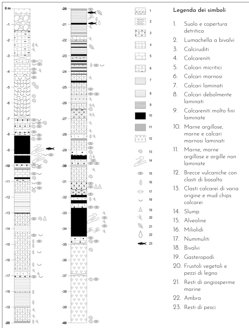
Log stratigrafico completo della successione recuperate nel carotaggio in Pesciara del 2015
