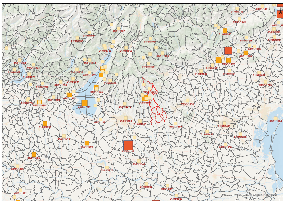
Mapa con l'ubicazione degli epicentri dei terremoti che hanno causato danni nell'area di candidatura e all'esterno della stessa
