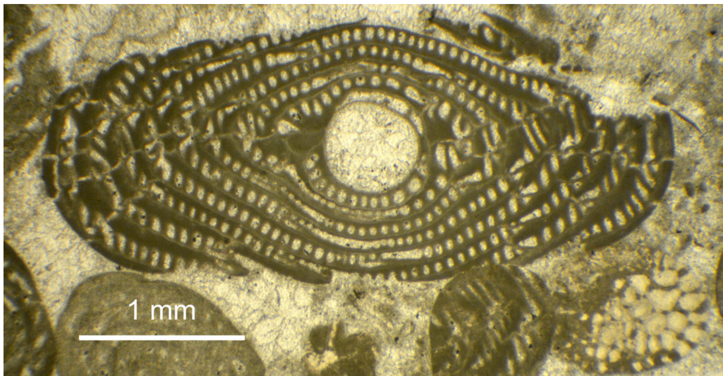
Alveolina postalensis in sezione sottile
