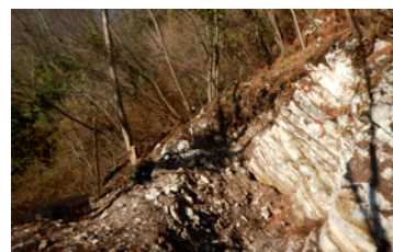
C. Affioramento sul Monte Postale
