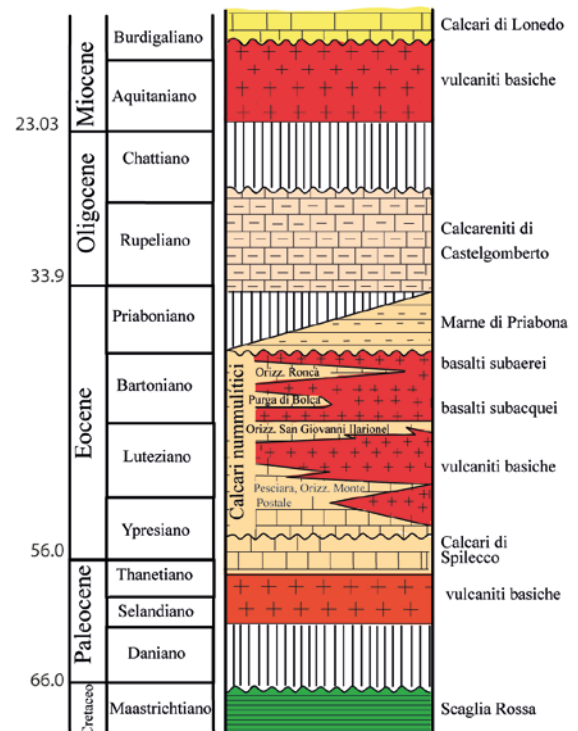
Colonna stratigrafica dei Monti Lessini orientali (da Brombin et al., 2019 - modificata)
