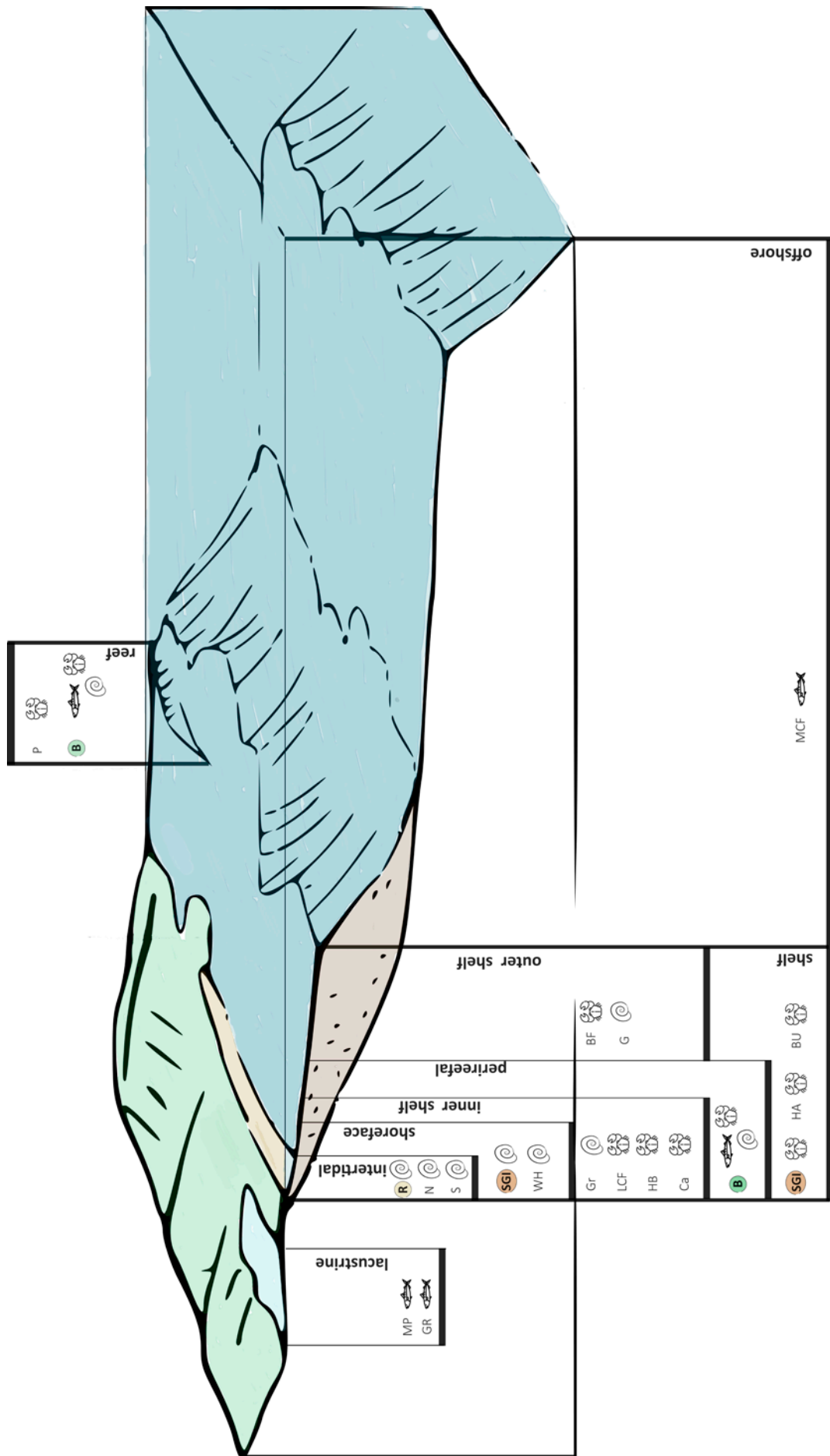
Modello rappresentativo dei diversi ambienti riferiti ai siti dell'Eocene su cui è stata fatta la comparazione.
