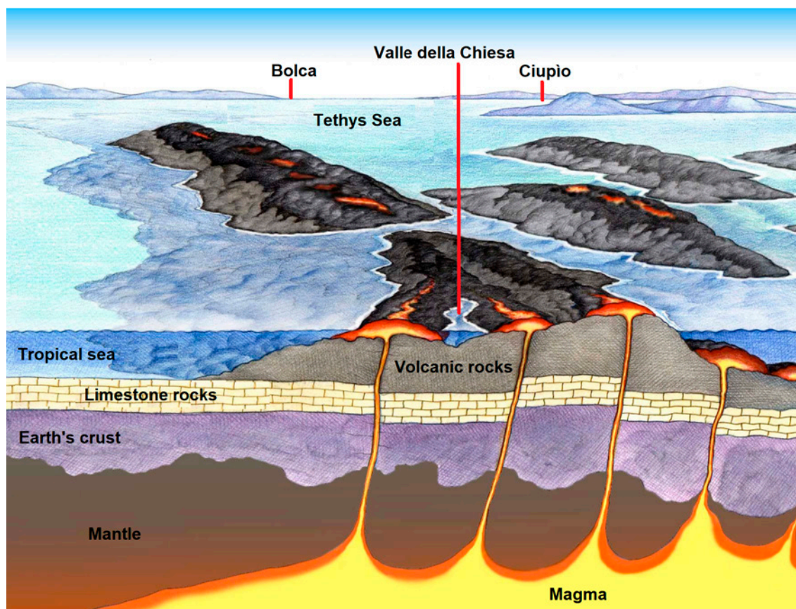
Ricostruzione paleogeografica del territorio di Ronca durante l'Eocene
