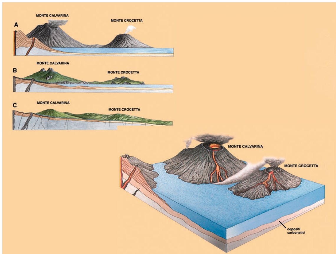
Evoluzione morfologica dall'Eocene ai giorni nostri dei due principali edifici vulcanici della Val d'Alpone
