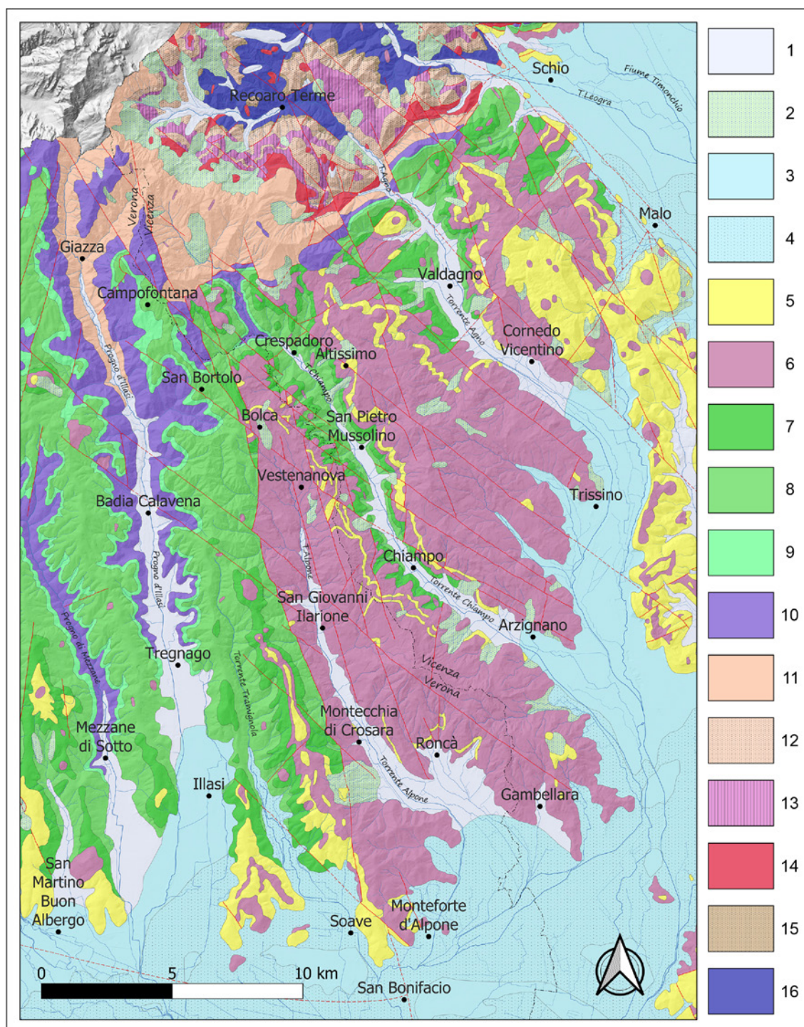
Carta geologica dell'area di candidature e del territorio circostante
