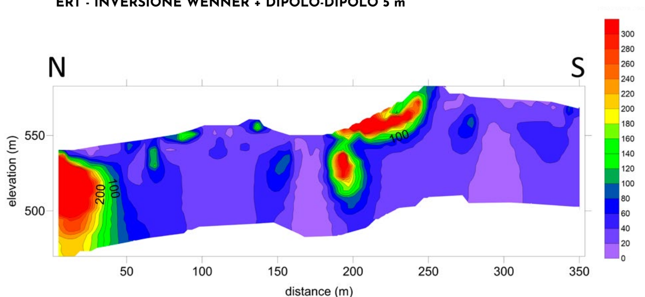
Profilo geoelettrico nell'area della Pesciara
