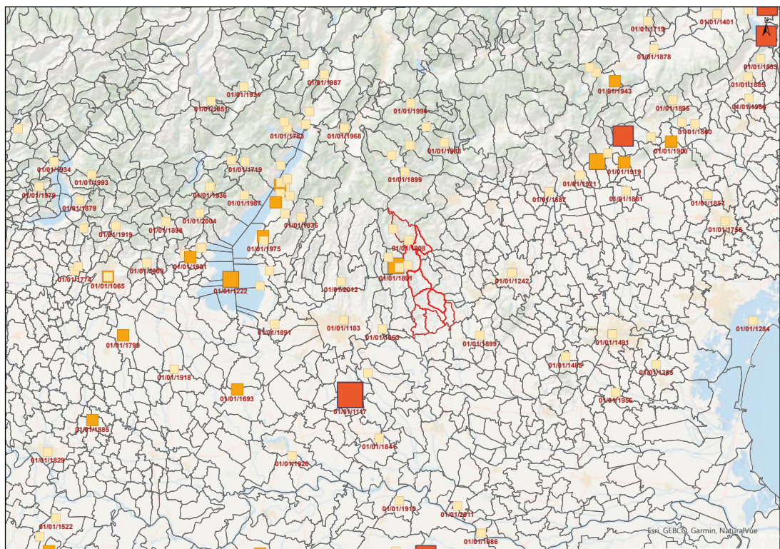
Mappa con l'ubicazione degli epicentri dei terremoti che hanno causato danni nell'area di candidatura e all'esterno della stessa
